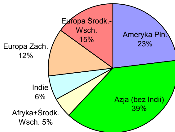
Światowe zdolności produkcyjne sody kalcynowanej (2007r. - 55 mln ton)
